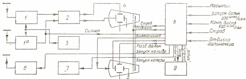
Рис. 3. Упрощенная блок-схема „круга“. 1 — приемные устройства; 2 — фазовые развертки; 3 — гетеродин; 4 — электронно-лучевые трубки фазометра (8ЛО-29); 5 — электронно-лучевая трубка дальнотмера (8ЛО-30); 6 — фоторегистрирующая камера КС-50Б; 7 — передатчик сигналов калибровки; 8 — синхронизирующий блок шкафа; 9 — дискриминатор.
