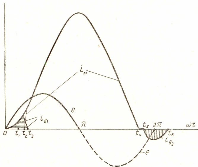
Рис. 3. Величина тока в различных элементах схемы: i_{\delta 1} —ток через вентиль B_1 , i_m —ток через механический контактный аппарат, i_{\delta 2} —ток через вентиль B_2 .
