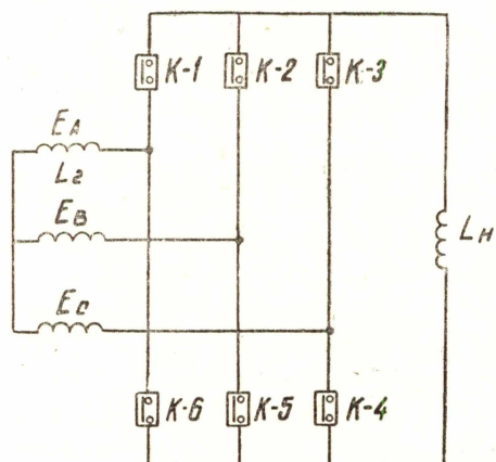
Рис. 1. Принципиальная схема включения генератора на нагрузку.
