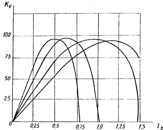
Рис. 4. Коэффициент усиления при отсутствии обратной связи. Выпрямитель ротора собран по трехфазной однополупериодной схеме.
