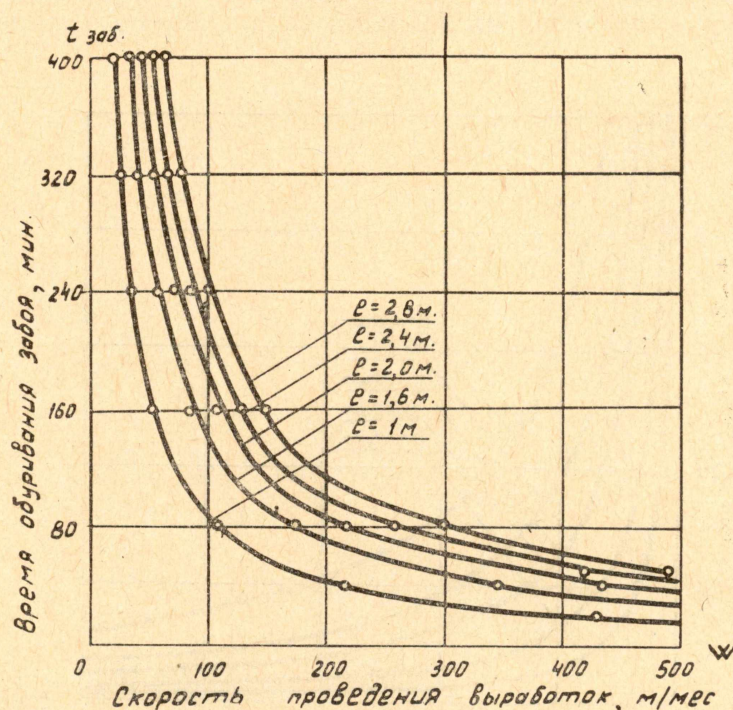
Рис. 4. Влияние производительности бурильной машины и числа шпуров на время обуривания забоя
