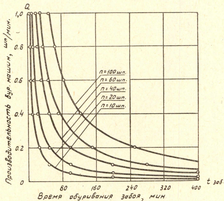
Рис. 5. Влияние времени обуривания забоя и глубины шпуров на скорость проведения выработок
