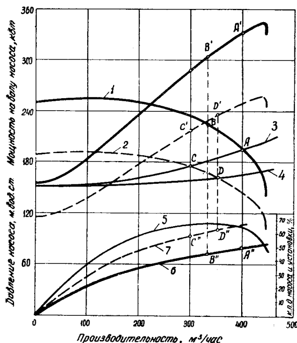
Рис. 2. Характеристика водоотливной установки с насосом типа АЯПЗ-300.
