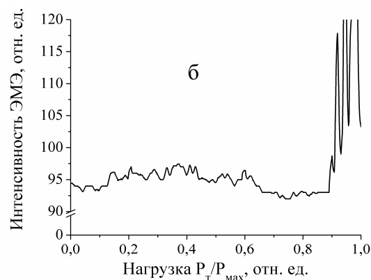
Рис. 3. Изменения: а) тока поляризации i_p и б) электромагнитной эмиссии при нагружении до разрушающих значений P_{max} образца эпидот-гранатового скарна
