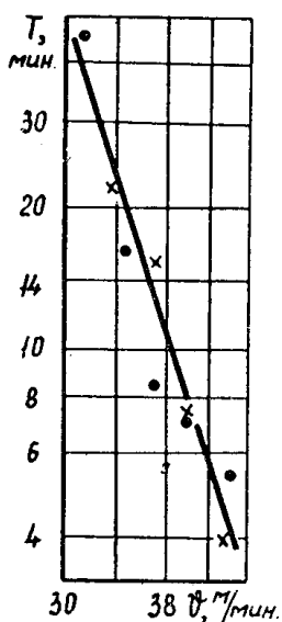
Рис. 1. Зависимость времени стойкости резцов T от скорости резания V при различных режимах трехкратных отпусков. ● — обычный отпуск при 560°, × — кратковременный отпуск при 600°
