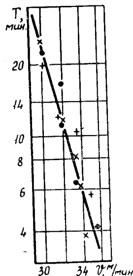
Рис. 2. Зависимость времени стойкости резцов T от скорости резания V при различных режимах отпуска. ● — трехкратный отпуск при 560°, × — трехкратный отпуск при 600°, + — двухкратный отпуск при 600°
