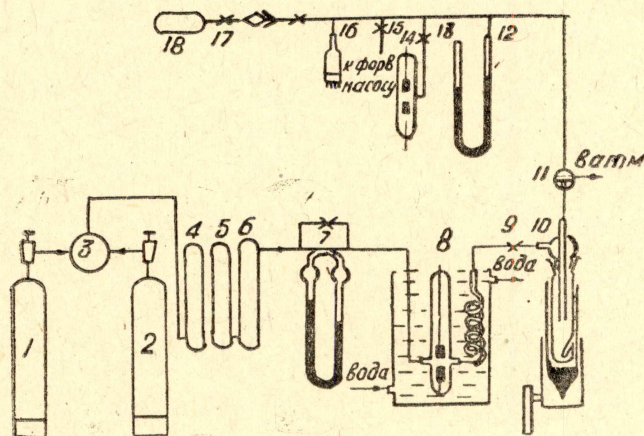
Рис. 1. Схема установки.
