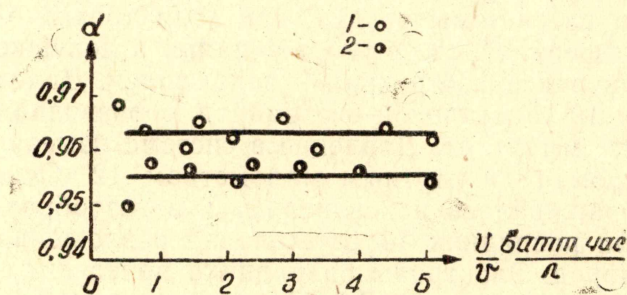
Рис. 3. Зависимость коэффициента разделения от удельной энергии разряда. 1 — коэффициент разделения для азота, 2 — коэффициент разделения для кислорода.
