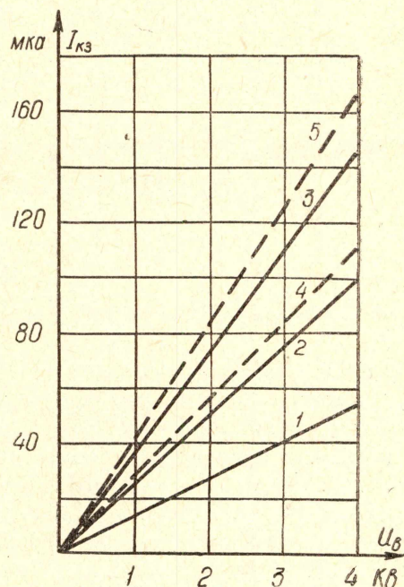
Рис. 2. График зависимостей I=f(U_v) , снятых по схемам рис. 1. Опытные: 1) при p=1 , 2) при p=2 , 3) при p=3 ; расчетные: 4) при p=2 , 5) при p=3 .
