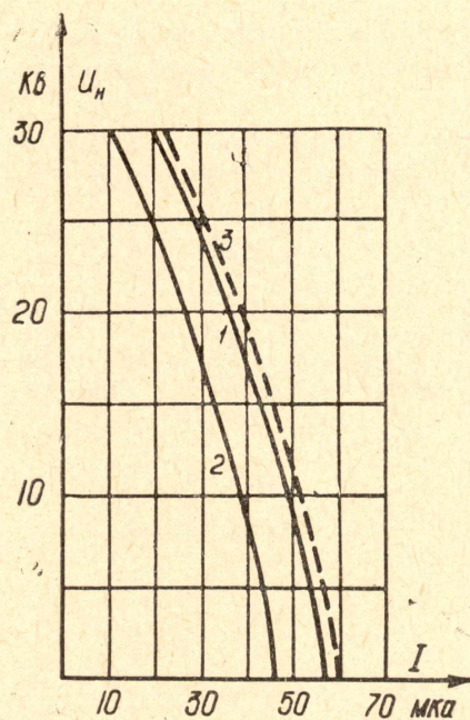
Рис. 4. График зависимости U_H = f(I_H) : 1) при независимой работе одной пары полюсов, 2) при работе многополюсного генератора с одинаковой полярностью возбуждения, 3) при работе многополюсного генератора с разной полярностью возбуждения.
