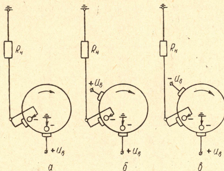
Рис. 3. Схемы соединения ЭСГ: а) независимая схема одной пары полюсов, б) схема с одинаковой полярностью возбуждения, в) схема с разной полярностью возбуждения.
