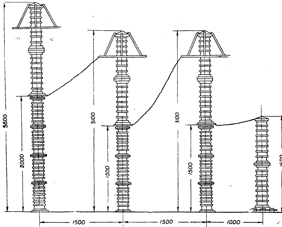
Рис. 2. Разрядник РВС-220 в исполнении из 4-х колонн (вариант 3).
