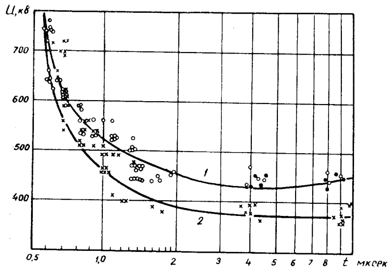
Рис. 3. Вольтсекундные характеристики разрядника РВС-220 в заводском исполнении: 1 — экранное кольцо D = 1880 мм с глубиной посадки 1200 мм; 2 — то же с глубиной посадки 900 мм. X X — отрицательный импульс напряжения, O O — положительный импульс напряжения.
