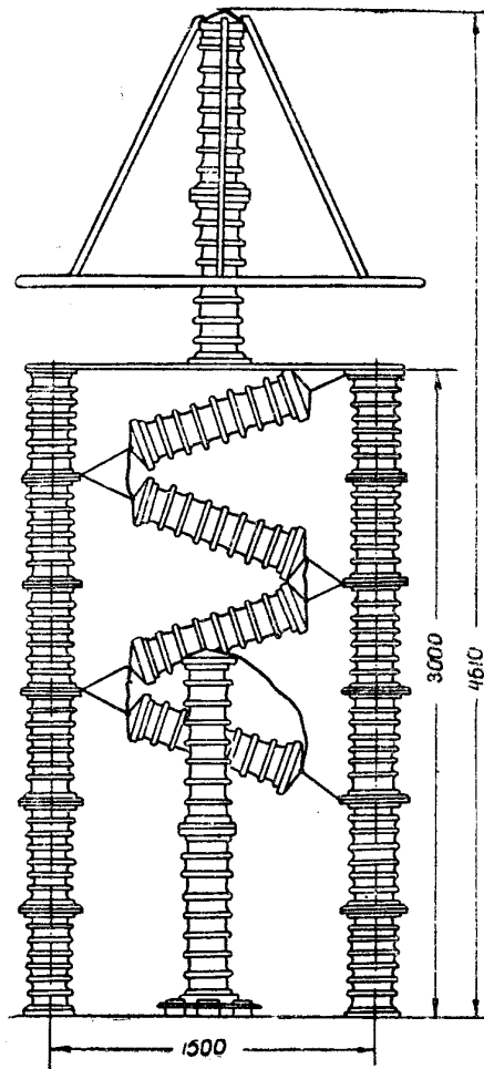
Рис. 1. Разрядник РВС-220 в исполнении на двух опорных колоннах из изоляторов КО — 400 (вариант 2).
