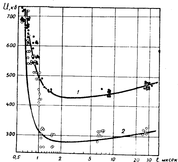
Рис. 4. Вольтсекундные характеристики РВС-220 в варианте 2: 1 — нормальное кольцо D = 1880 мм, глубина посадки 1200 мм; 2 — то же с глубиной посадки 900 мм.
