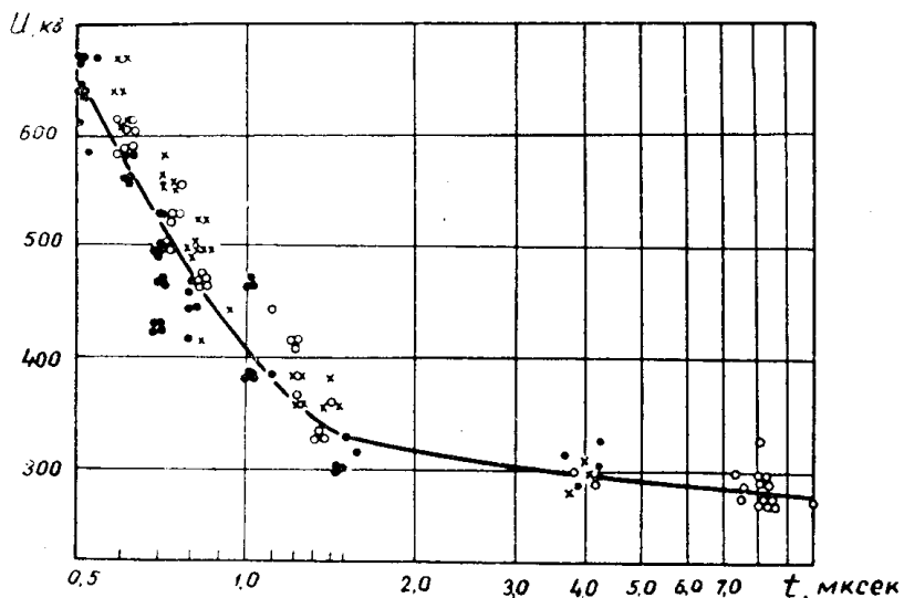
Рис. 5. Вольтсекундная характеристика разрядника РВС-220 в исполнении по варианту 3.
