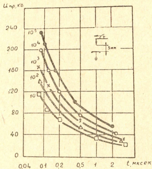
Рис. 1. Вольтсекундные характеристики водных растворов при вероятности пробоя \psi = 5\% и положительной полярности „стержня“.
