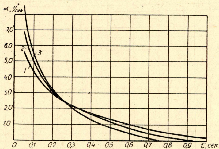
Рис. 3. Изменение константы скорости горения Назаровского бурого угля по времени выгорания. 1 — при 700°C; 2 — при 720°C; 3 — при 747°C.
