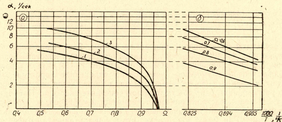
Рис. 4. Зависимость константы скорости горения Назаровского бурого угля от степени выгорания (а) и температуры (б). 1, 2, 3 — то же, что на рис. 3.
