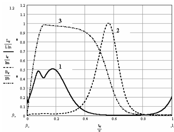
Рис. 2. Относительные временные зависимости изменения: 1) индуктивности обмотки, 2) генерируемого тока и 3) индукции в статоре генератора
