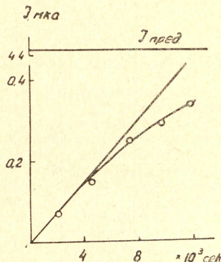
Рис. 2. Зависимость глубины анодного зубца урана от времени электролиза ( C = 1 \cdot 10^{-8} г-ион/л; 2N серная кислота; t = 19^\circ C ; пленочный электрод).
