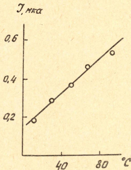
Рис. 4. Влияние температуры на анодный зубец урана ( C = 2,5 \cdot 10^{-8} г-ион/л; \tau_э = 10 мин; 26 N серная кислота; пленочный электрод).
