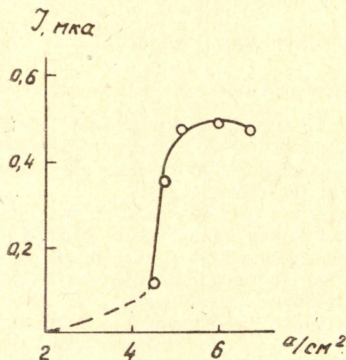
Рис. 1. Зависимость глубины анодного зубца урана от плотности тока электролиза (фон — 1,8N H_2SO_4 ; \tau_0 = 10 мин; t = 20^\circ C ; C = 0,5 \cdot 10^{-6} г-ион/л; пленочный электрод).
