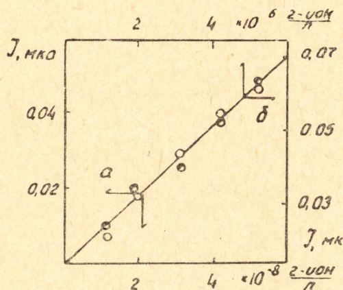
Рис. 3. Зависимость глубины анодного зубца урана от концентрации урана в растворе (2 N серная кислота, \tau_э = 10 мин; T = 23^\circ\text{C} ): а) пленочный электрод — \circ , б) ртутная капля — \bullet .
