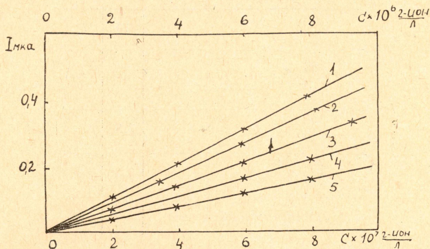
Рис. 3. Зависимость глубины анодных зубцов элементов от концентрации ионов металла в растворе 1%-ный оксихинолин в \text{CHCl}_3 + 0,2N \text{ NH}_4\text{NO}_3 в \text{CH}_3\text{OH} (1:1): 1 — свинец; 2 — кадмий, 3 — индий, 4 — медь, 5 — таллий. Условия опытов: чувств. 1 : 10^{-8} а/мм; потенциал электролиза \varphi_э = -1,2 в, время электролиза \tau_э = 5 мин.
