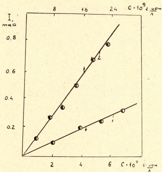
Рис. 5. Зависимость глубины анодных зубцов свинца от концентрации ионов металла в растворе: 1. чув. 1 : 10^{-8} а/мм, \tau_э = 5 мин; \varphi_э = -1,0 в; T = 25^\circ\text{C} ; при использовании эффекта амальгамы аммония и повышенной температуры; чув. 1 : 10^{-8} а/мм; \varphi_э = -2,85 (в); \tau_э = 5 мин; T = 80^\circ\text{C} .
