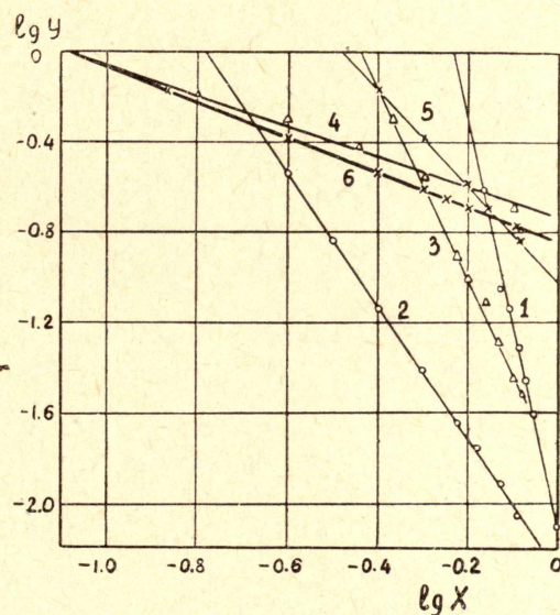
Рис. 1. График зависимости \lg y - \lg x C_{2G1} - aAu_n C_{Ga} \cdot 10^{+4} г-ион/л (1) — — 1,0; (2) — 2,0; (3,4) — Ga Co_n C_{Ga} \cdot 10^{+4} г-ион/л (3) — 1, 0; (4) — 2,0 5,6) — Ga Ni_n C_{Ga} \cdot 10^{+4} г-ион/л (5) — — 1, 0; (6) — 1,6
