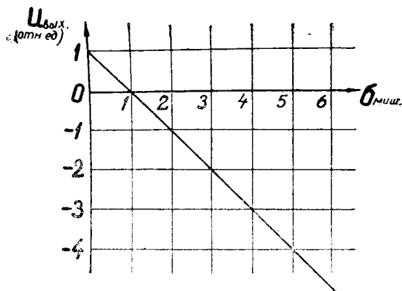
Рис. 2. Зависимость величины выходного напряжения преобразователя от коэффициента вторичной эмиссии мишени.
