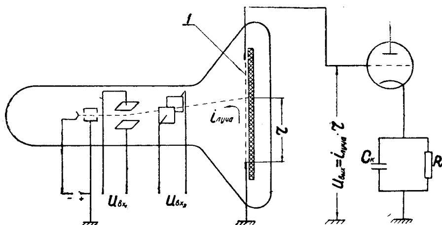
Рис. 1. Схема включения электронно-лучевого функционального преобразователя. 1—проводящий слой мишени.
