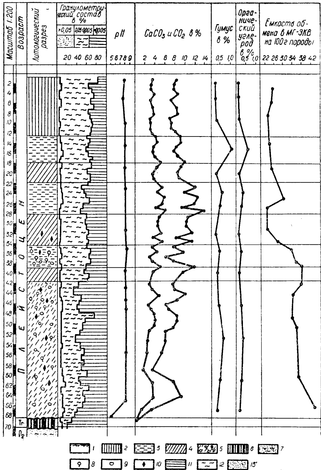
Рис. 1. Литологический разрез и отдельные показатели грансостава и химических свойств четвертичных отложений северо-западной части Присалаирской депрессии по скв. 314: 1 — современная почва; 2 — лёссовидные тяжелые суглинки и глины; 3 — глины грязно-серые иловатые; 4 — глины серовато-бурые; 5 — глины коричневые, темно-коричневые и др. 6 — глины пестроцветные; 7 — алевролиты тонкослоистые светло-серой окраски; 8 — обломки раковин остракод; 9 — обломки пород; 10 — известковистые новообразования; 11 — глинистая фракция (< 0,005 мм) в %; 12 — пылеватая фракция (0,05—0,005 мм) в %; 13 — песчаная фракция (> 0,05мм) в %.
