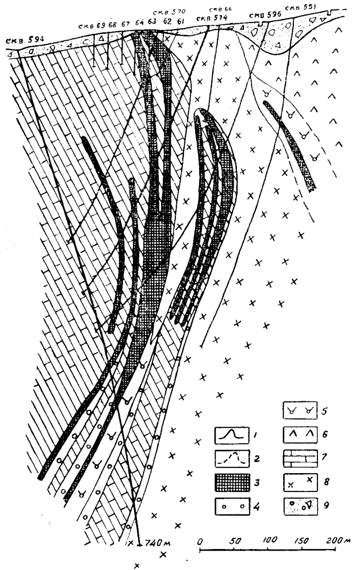
Рис. 2. Разрез через рудное тело IX и рудную зону XII по последним данным. 1 — наблюдаемая кривая вертикальной составляющей магнитного поля, 2 — теоретическая кривая от разреза, 3 — руды, 4 — скарны, 5 — альбитофиры, 6 — амфиболиты, 7 — известняки, 8 — диориты, 9 — делювий.
