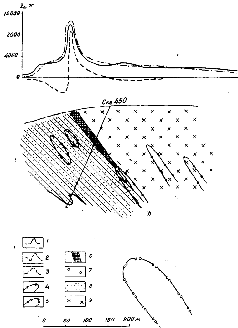
Рис. 3. Разрез через рудное тело XIV в районе слабой магнитной аномалии. 1 — наблюдаемая кривая вертикальной составляющей магнитного поля, 2 — теоретическая кривая от известного рудного тела, 3 — теоретическая кривая от известного тела и от предполагаемых дополнительных рудных тел, 4 — контуры предполагаемых дополнительных рудных тел по варианту с наименьшими возможными глубинами, 5 — контуры предполагаемого рудного тела по варианту с одним глубоко залегающим рудным телом, от которого теоретическое поле на поверхности составит 2000—2500 гамм вблизи эпицентра, 6 — руды, 7 — скарны, 8 — песчаники, 9 — диориты.
