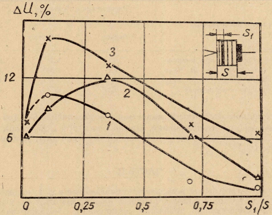
Рис. 2. Влияние положения барьера на пробивное напряжение пакета кабельной бумаги. Импульсы положительной полярности, \tau_{фр} = 10^{-5} сек. Материал барьера: 1 — полиэтилен, 2 — фторопласт-4, 3 — полистирол.
