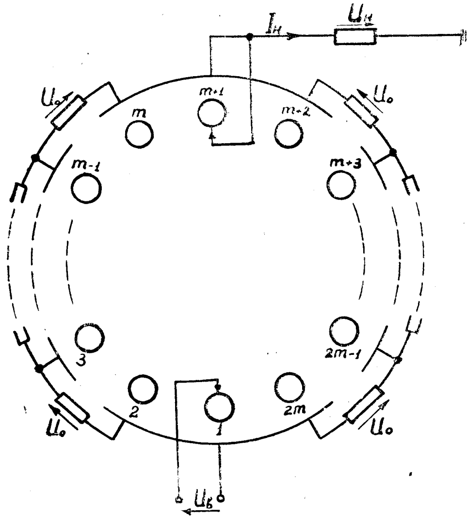
Рис. 1. Принципиальная схема ЭСГ с каскадным соединением транспортеров-проводников.
