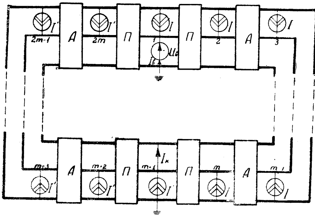
Рис. 3. Расчетная цепная схема.
