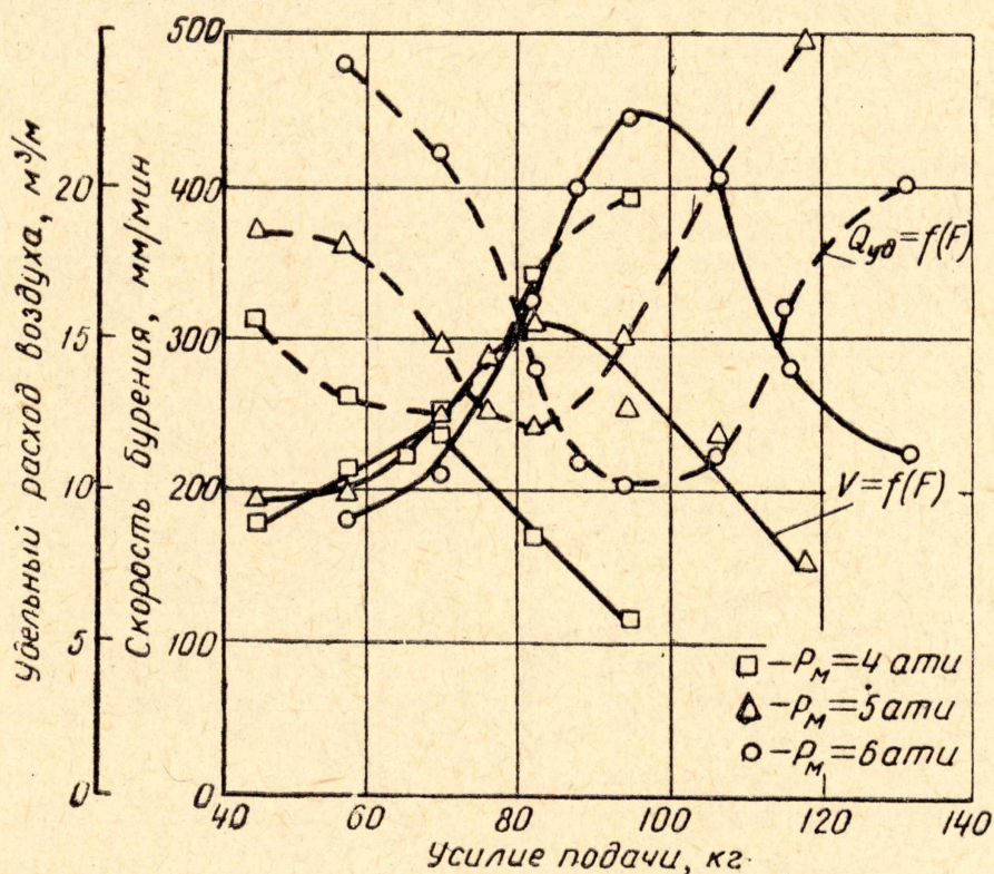
Рис. 4. Зависимость скорости бурения и удельного расхода воздуха от усилия подачи при бурении песчаника ( f=6 \div 8 ) молотком ПР-20.
