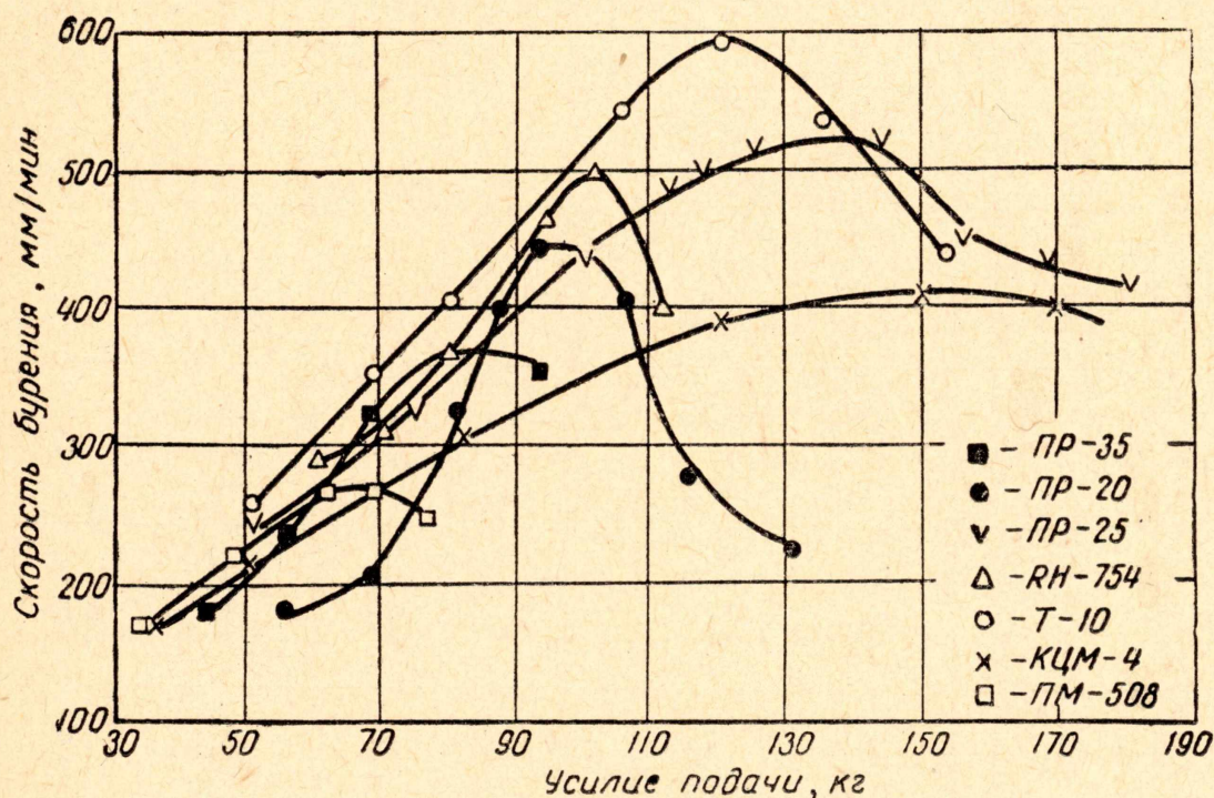
Рис. 1. Зависимость скорости бурения песчаника ( f=6 \div 8 ) от усилия подачи при давлении воздуха 6 атм.
