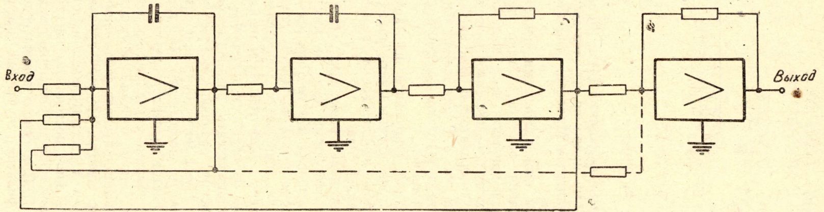
Рис. 3. Схема набора фильтров на решающих усилителях
