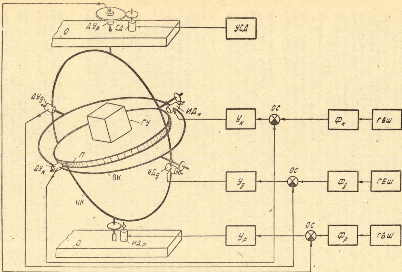
Рис. 4. Схема стенда для испытаний бортовых гироскопических устройств в режиме случайной качки
