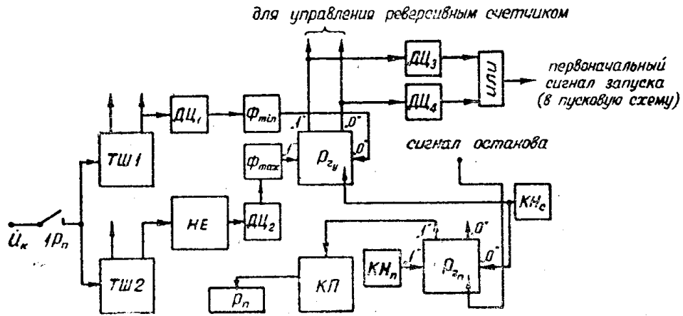
Рис. 1. Функциональная схема блока экстремумов, пуска и останова
