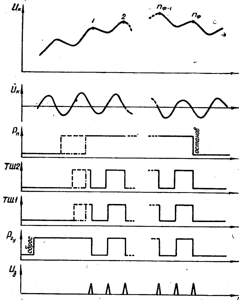
Рис. 2. Временные диаграммы блока экстремумов, пуска и останова
