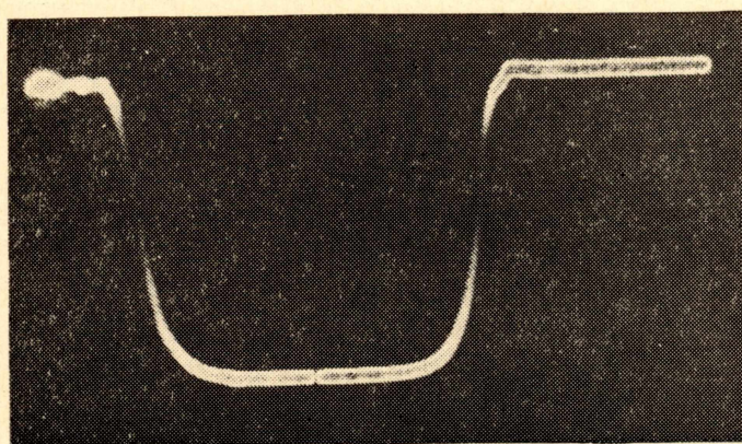
Рис. 3. Осциллограмма тока ускорительной трубки
