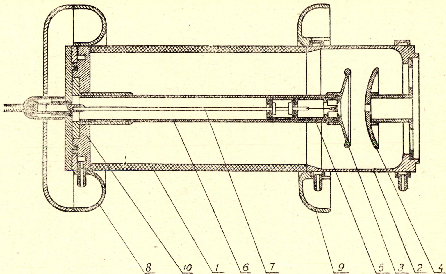
Рис. 1. Конструкция ускорительной трубки: 1 — фарфоровый цилиндр; 2 — стальной цилиндр; 3 — катодный электрод; 4 — анод; 5 — катодный блок; 6 — труба; 7 — стержень; 8 и 9 — экраны; 10 — катодный фланец
