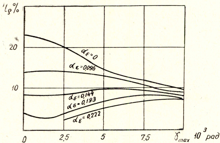
Рис. 2. Коэффициент захвата на первом этапе инъекции. Изменение магнитного поля \dot{H} = 90 кгс/сек в сек
