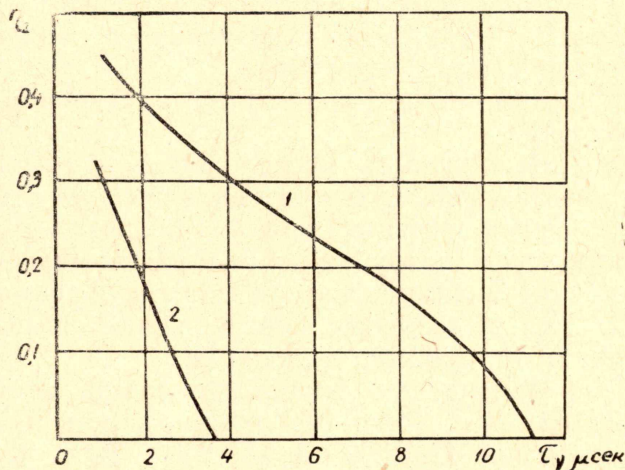
Рис. 5. Коэффициент захвата на втором этапе инжекции
