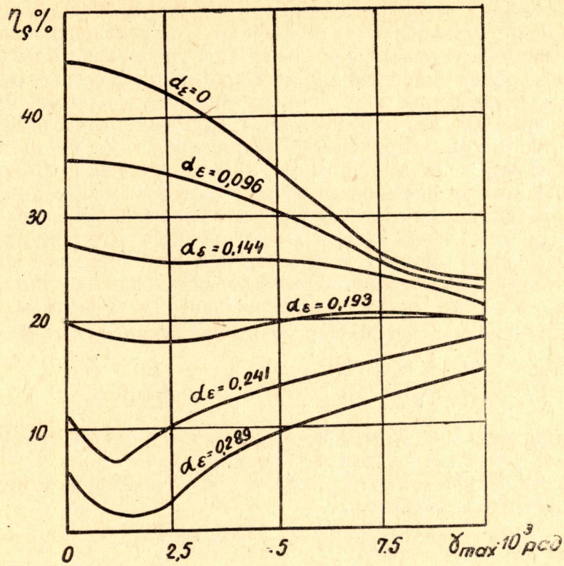
Рис. 3. То же, что и на рис. 2, но для \dot{H} = 175 кг/сек в сек
