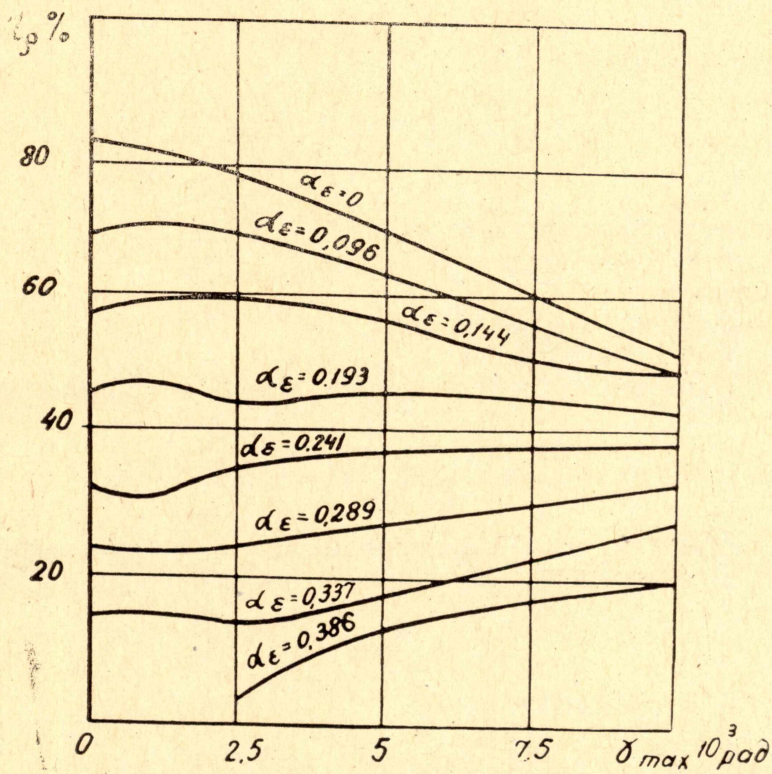
Рис. 4. То же, что и на рис. 2, но для \dot{H} = 300 кг/сек в сек
