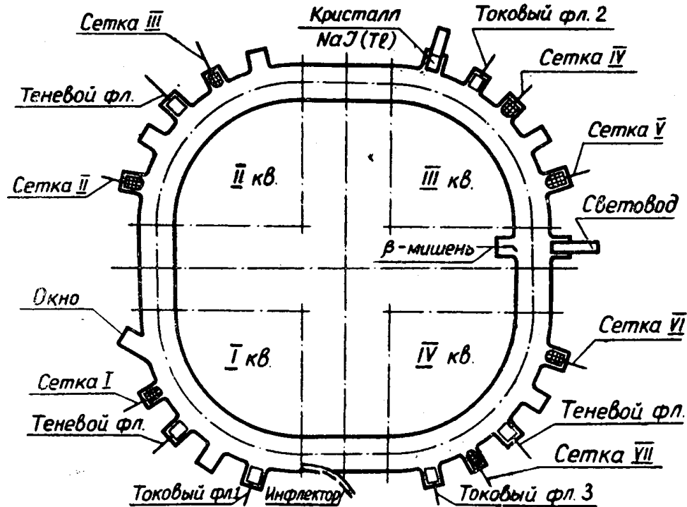
Рис. 1. Размещение элементов системы индикации в камере синхротрона
