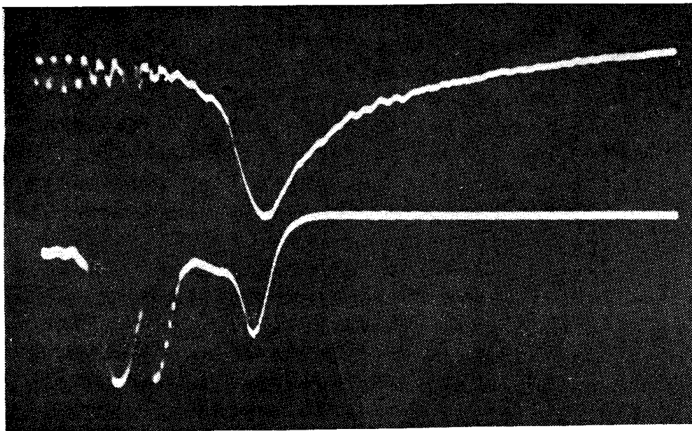
Рис. 3. Осциллограммы импульсов квазибетатронного режима ускорения (верхний импульс — с \beta -мишени с ФЭУ-11Б, нижний импульс — со схемы с кристаллом)
