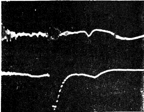
Рис. 2. Осциллограммы импульсов квазибетатронного режима ускорения (верхний импульс — с токовой \beta -мишени, нижний импульс — со схемы с кристаллом)
