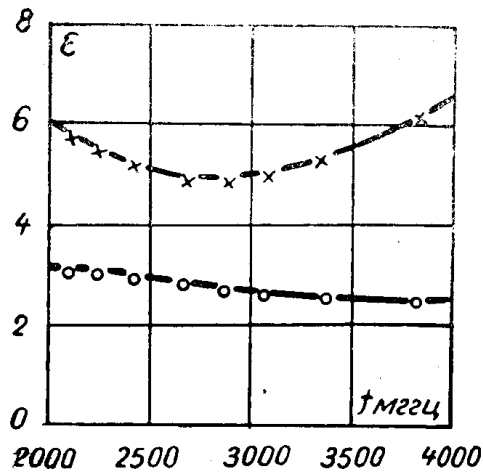
Рис. 2. Зависимость проницаемости от частоты. ○ — оргстекло, × — гетинакс
