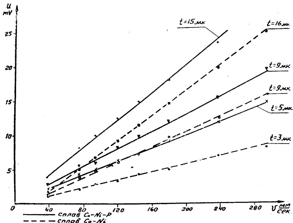
Рис. 1 Влияние толщины покрытия и состава сплава на величину снимаемого сигнала.
