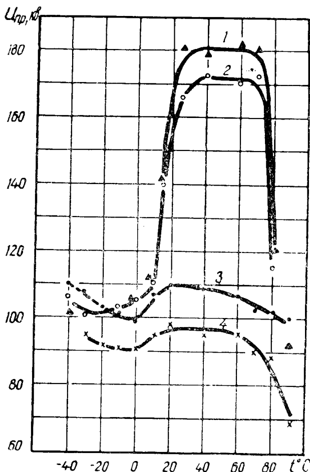
Рис. 2 Температурные зависимости импульсных пробивных напряжений полиэтилена высокой и низкой плотности при различных крутизнах фронта. 1 — полиэтилен высокой плотности, a = 500 кВ/мксек, 2 — полиэтилен низкой плотности, a = 500 кВ/мксек, 3 — полиэтилен высокой плотности, a = 30 кВ/мксек, 4 — полиэтилен низкой плотности, a = 30 кВ/мксек.
