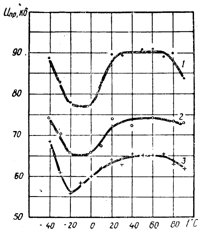
Рис. 1 Температурные зависимости импульсных пробивных напряжений политетрафторэтилена при различных крутизнах фронта. 1— a=500 кВ/мксек; 2— a=250 кВ/мксек; 3— a=30 кВ/мксек.
