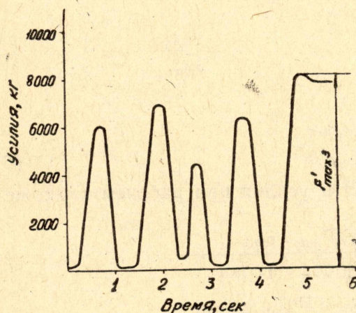
Рис. 3. Диаграмма усилий в тормозной тяге при рабочем торможении (Восточный скиповый подъем шахты 9-15, треста «Анжероуголь»)
