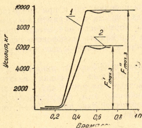
Рис. 5. Диаграммы усилий в тормозных тягах скиповой подъемной машины шахты «Зиминка — Капитальная» треста «Прокопьевскуголь»: 1 — верхняя горизонтальная тяга; 2 — нижняя горизонтальная тяга
