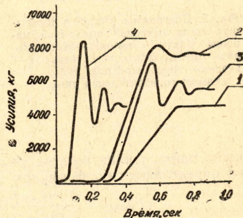
Рис. 4. Диаграммы усилий в тормозных тягах при предохранительном торможении: 1 — скиповый подъем рудника Салаир; 2 — скиповый подъем рудника Таштагол; 3 — скиповый подъем шахты «Дальние Горы» треста «Киселевскуголь»; 4 — лабораторная подъемная установка.
