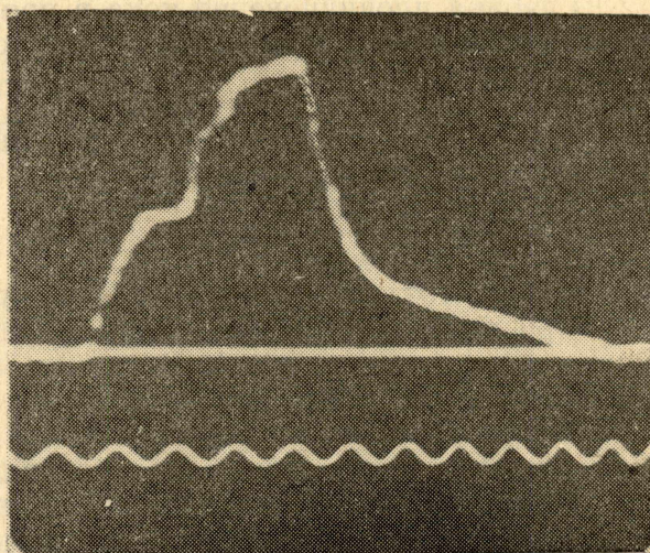
Рис. 3. Осциллограмма пробоя.
