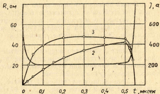
Рис. 2. Влияние параметров контура R, L, C на время нарастания и время спада тока при заданном изменении активного сопротивления от времени: 1 — R(t) ; 2 I(t) при L=5 мкГн, C=1 мкФ; 3 — I(t) при L=1 мкГн, C=1 мкФ.
