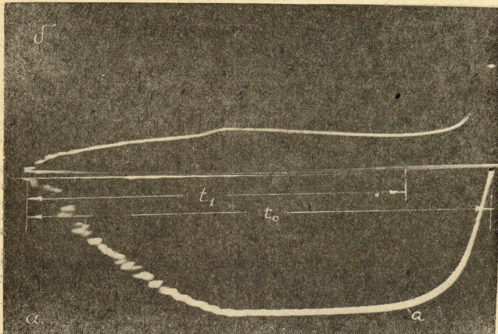
Рис. 1. Осциллограммы тока (а) и напряжения (б) при взрыве проволочки.
