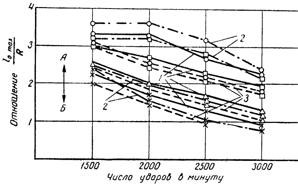
Рис. 5. Зависимость отношения \frac{l_{\max}}{R} от числа ударов:
