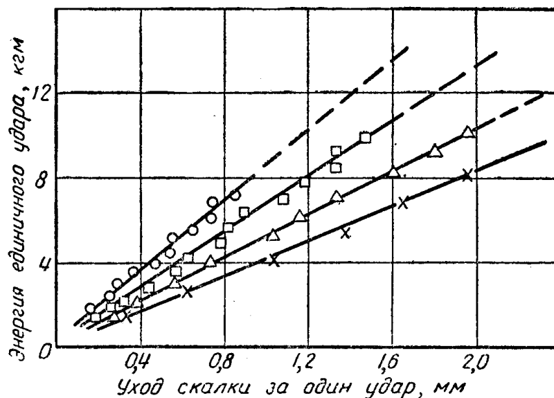
Рис. 2. Зависимость ухода скалки от энергии единичного удара:
