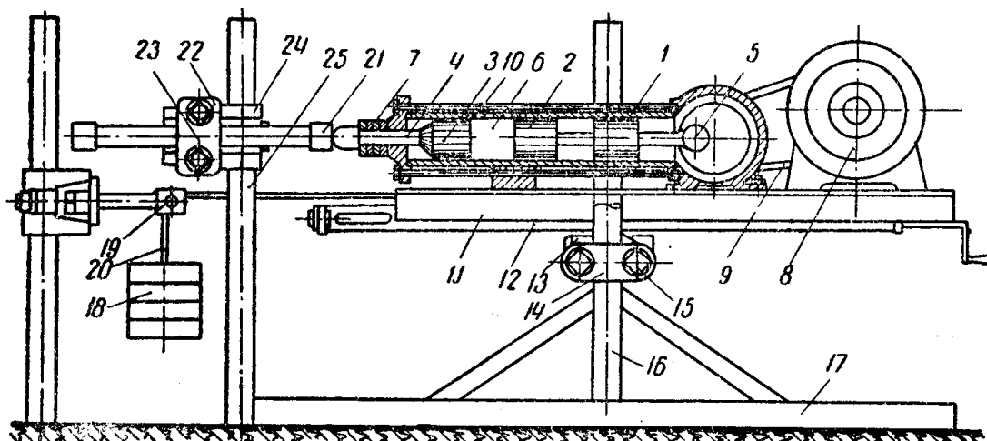
Рис. 1. Общий вид экспериментальной установки.
