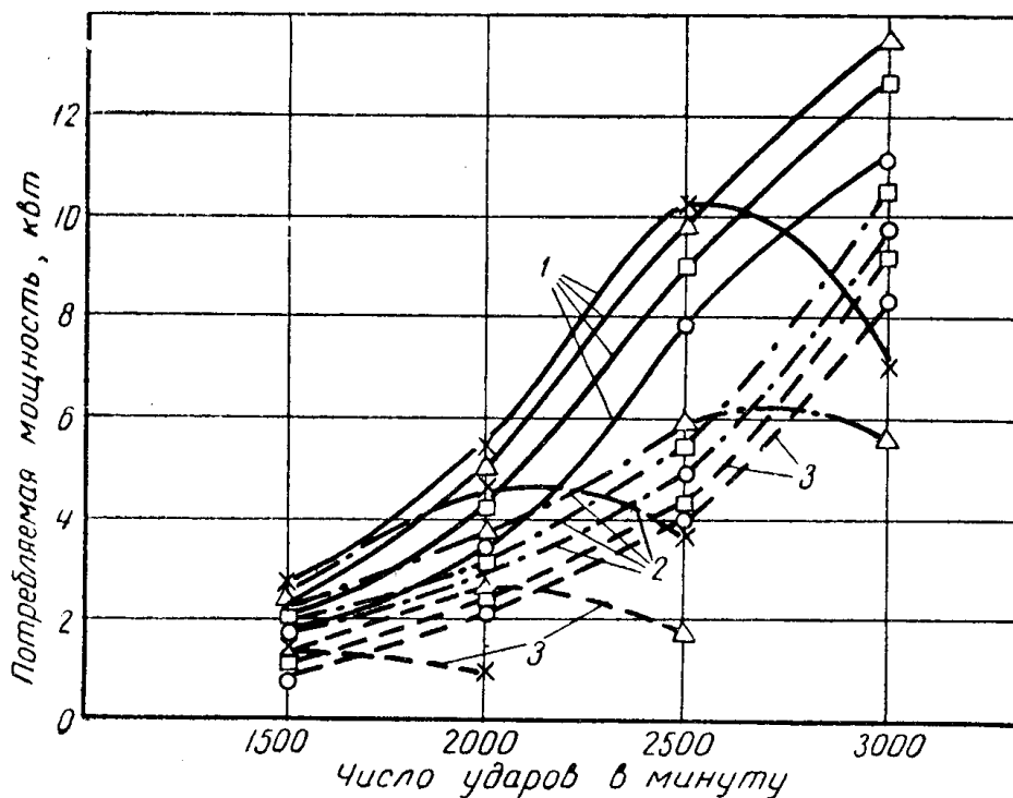
Рис. 7. Зависимость потребляемой мощности от числа ударов: ○ — Q_6 = 0,55 кг; □ — Q_6 = 0,70 кг; △ — Q_6 = 1,0 кг; × — Q_6 = 1,35 кг; 1 — R = 30 мм; 2 — R = 25 мм; 3 — R = 20 мм.
