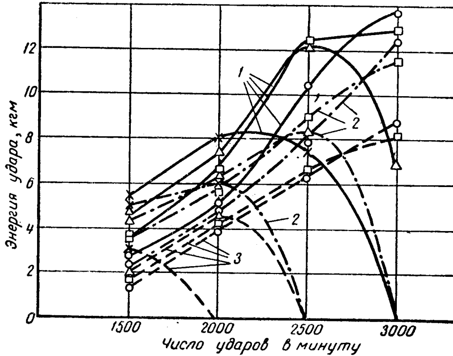
Рис. 6. Зависимость энергии удара от числа ударов:
