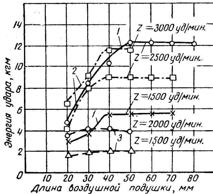
Рис. 4. Зависимость энергии удара от длины воздушной подушки:
