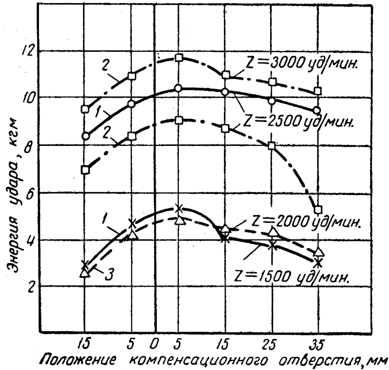
Рис. 3. Зависимость энергии удара от положения компенсационного отверстия:
