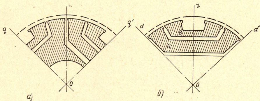
Рис. 2. Форма моделей электродов при моделировании магнитного поля:
