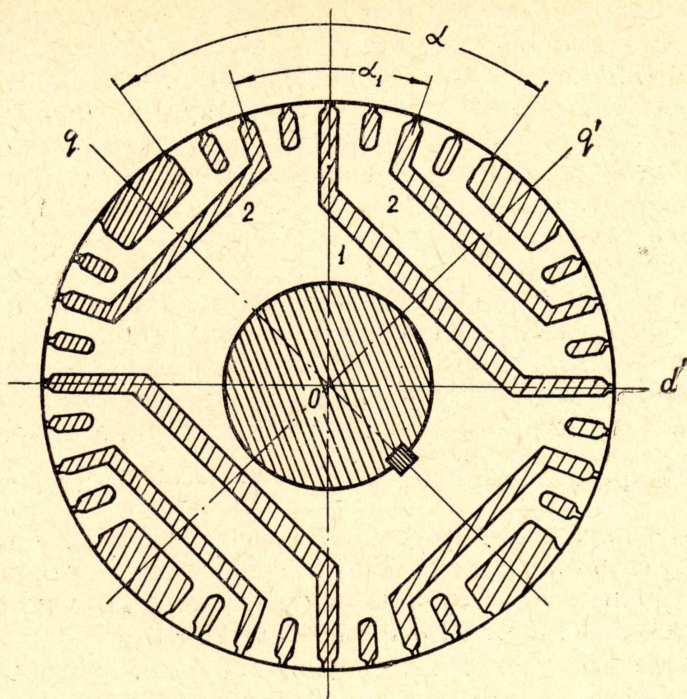
Рис. 1. Поперечный разрез ротора усовершенствованной СРМ.
