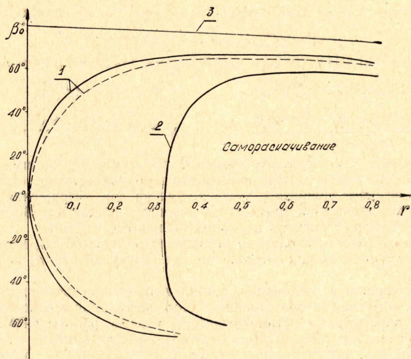
Р и с. 3. Границы области устойчивой работы, построенные в зависимости от угла нагрузки \beta_0 1 — T_d = 40 эл. сек, T_q = 0 ; 2 — T_d = 40 эл. сек, T_q = 10 эл. сек; 3 — граница сползания; — — — без учета переходных процессов с обмотки статора.
