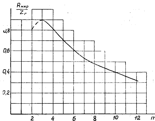
Рис. 3. Зависимость \frac{R_{нкp}}{Z_r} от числа фаз.
