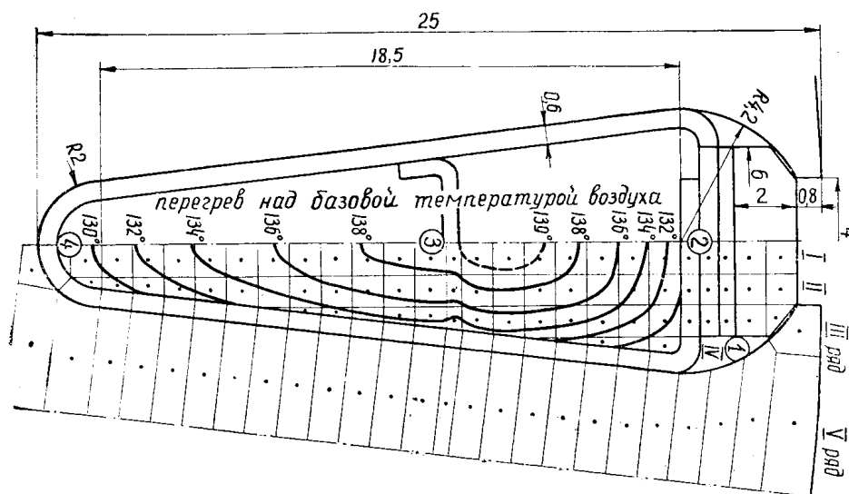
Рис. 1. Расчет температурного поля в пазу методом ячеек. 1 — 4 — места закладки термопар.
