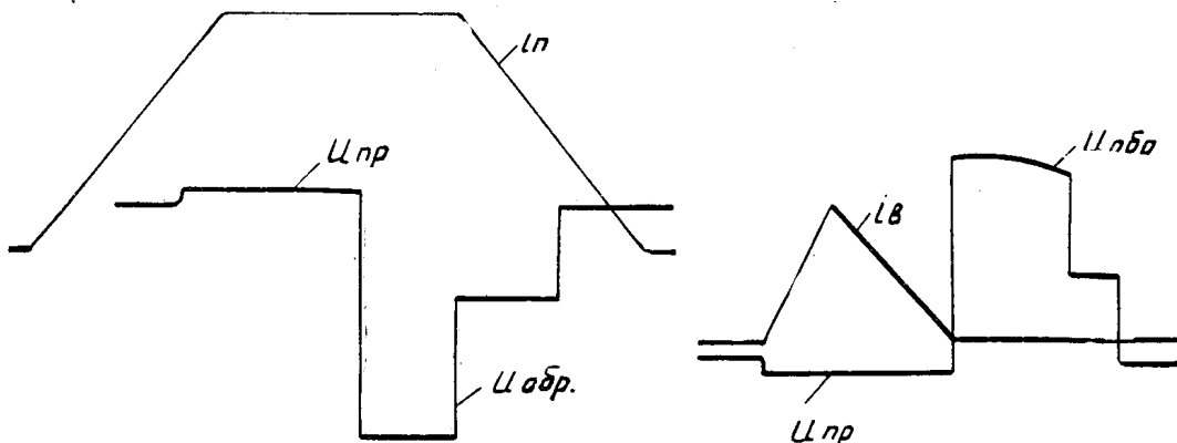
Рис. 2 б, в. Осциллограммы, снятые на экспериментальной машине.
