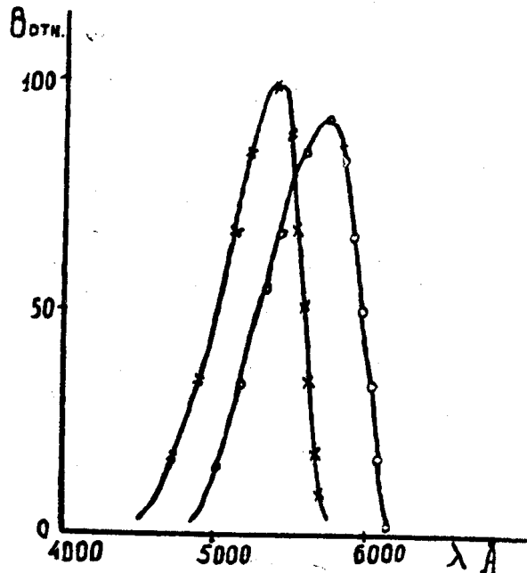
Рис. 2. Спектры свечения BaS — Mn-люминофоров при возбуждении переменным электрическим полем: ××× — зеленая полоса излучения ( \lambda_{\text{макс.}} = 5450 \text{ \AA} ); ○○○ — желтая полоса излучения ( \lambda_{\text{макс.}} = 5750 \text{ \AA} ).
