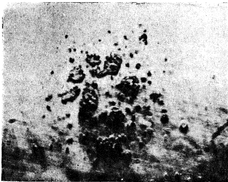
Рис. 3. Частицы молибдена, перенесенные незавершенным разрядом в 18 нсек на катод. Увеличение 800 \times
