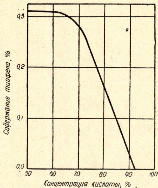
Рис. 1. Зависимость содержания тиофена в бензоле от концентрации серной кислоты. Соотношение БТК: \text{H}_2\text{SO}_4 + \text{CH}_2\text{O} = 100:2:1 . Время перемешивания с \text{H}_2\text{SO}_4 — 20 мин. Время перемешивания с \text{CH}_2\text{O} — 20 мин.
