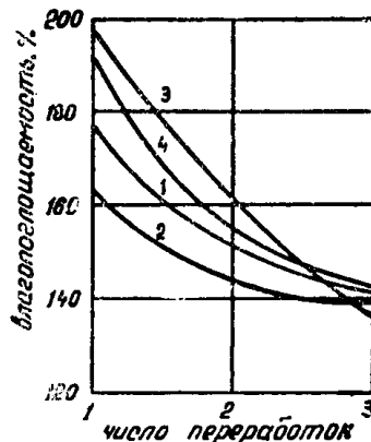
Рис. 3. Зависимость влагопоглощаемости формовок от степени переработки: 1 — формовки из торфа-сырца R = 45\% ; 2 — формовки из гидромассы R = 45\% ; 3 — формовки из торфа-сырца R = 35\% ; 4 — формовки из гидромассы R = 35\%
