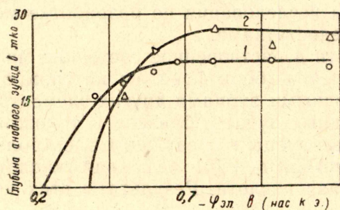
Рис. 1. Зависимость глубины анодных зубцов меди и свинца от потенциала электролиза на фоне \text{Ca Br}_2 + 0,5 N винная кислота. Кривая 1—для меди; кривая 2—для свинца. Условия опытов: 1. C=0,1 \gamma/\text{мл} \text{Cu} ; V=2,5 \text{мл} ; S=4 \cdot 10^{-9} \text{а/мм} ; \tau=10 \text{мин} ; r=0,04 \text{см} ; W=333 \text{мв'мин} . 2. C=0,1 \gamma/\text{мл} \text{Pb} ; V=3 \text{мл} ; S=8 \cdot 10^{-9} \text{а/мм} ; \tau=10 \text{мин} ; r=0,04 \text{см} .
