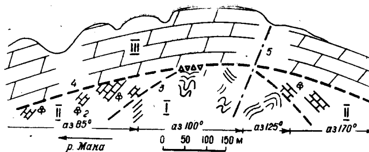
Рис. 2. Схематический разрез — зарисовка правого борта долины р. Маны сразу ниже Семенова утеса. I — слоистые темно-серые известняки анастасьинской толщи; II — темные и светлые массивные эпифитовые известняки верхов анастасьинской толщи; III — светлые массивные доломиты унгутской толщи; 1 — карбонатные брекчии в основании унгутской толщи; 2 — точки сборов флоры эпифитонов; 3 — согласная граница между слоистыми и массивными известняками анастасьинской толщи; 4 — граница углового несогласия между анастасьинской и унгутской толщами; 5 — тектоническое нарушение, осложняющее свод антиклинали
