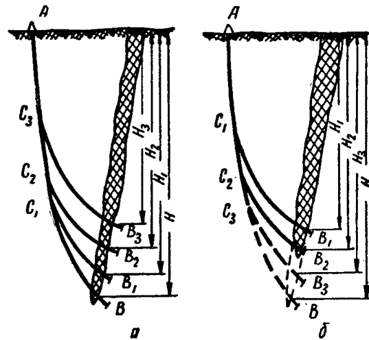
Рис. 1. Схема разведки многоствольными скважинами (по Б. И. Спиридонову): а — первая схема, б — вторая схема. AB — основной ствол; C_1B_1, C_2B_2, C_3B_3 — дополнительные стволы; H_1, H_2, H_3, H — вертикальные глубины подсечения полезного ископаемого.
