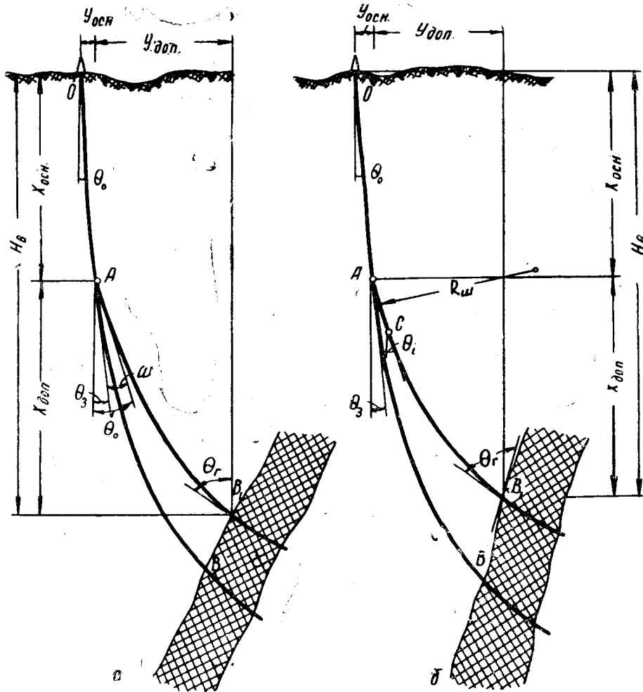
Рис. 2. Схемы многозабойных скважин: а — при отбуривании дополнительного ствола с помощью клина; б — при бесклиновом способе отбурки дополнительного ствола (с помощью одношарнирного отклонителя). H — глубина точки подсечения по вертикали; X_{осн} , X_{доп} и Y_{осн} , Y_{доп} — вертикальные и горизонтальные проекции участка OA основного ствола и дополнительного AB ; \Theta_3 , \Theta_i — зенитные углы в точке забурки дополнительного ствола, соответственно, у основного и дополнительного
