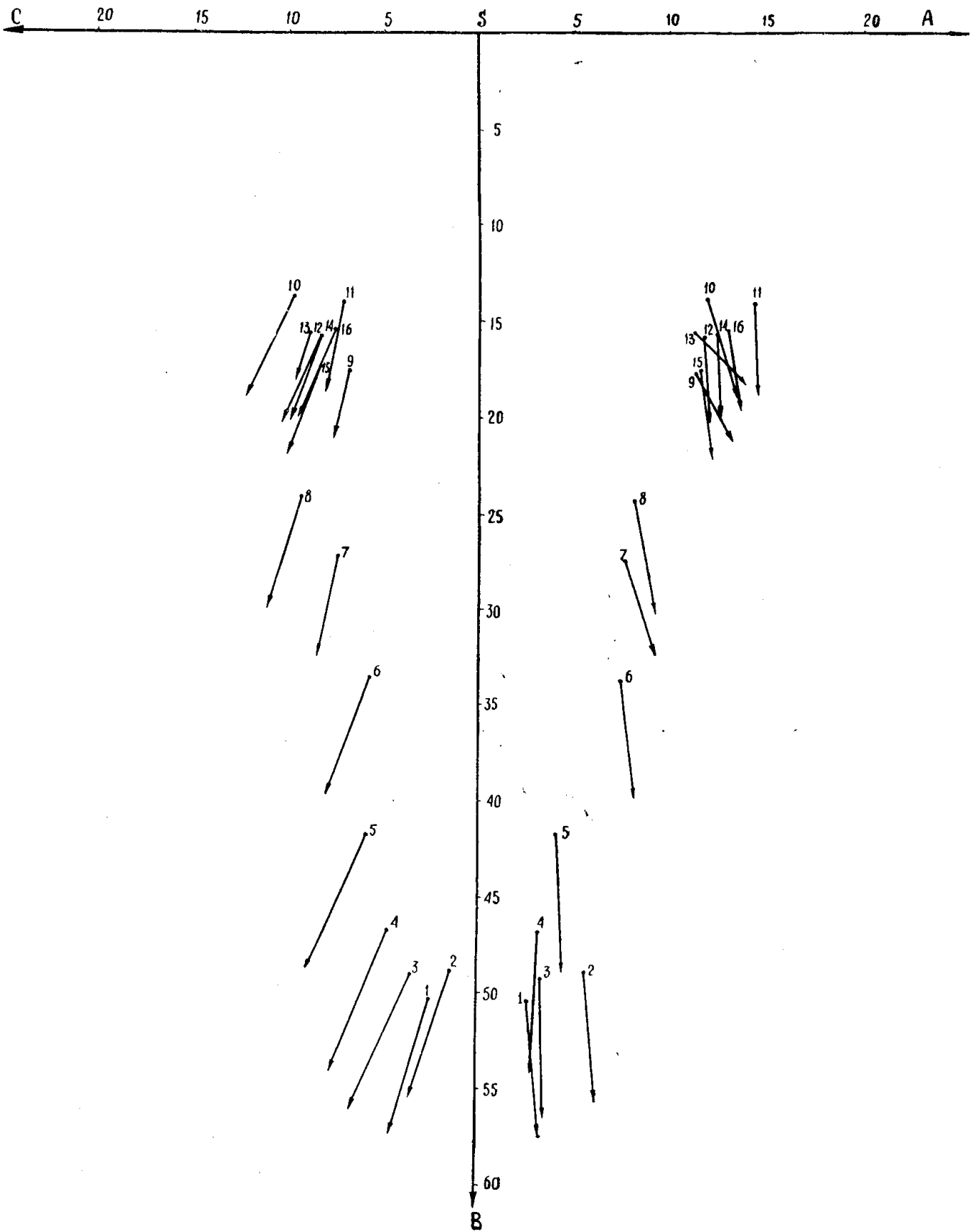
Рис. 1. Диаграмма химического состава пород Тилековского интрузивного комплекса (по А. Н. Заварицкому). 1, 2, 3, 4, 5 — верлиты; 6, 7, 8, 9, 10, 11 — переходные разности от верлитов к лейкократовым габбро, габбро-диабазам; 12, 13, 14, 15 — лейкократовое габбро, габбро-диабазы, 16 — лейкократовое габбро с щелочным уклоном.
