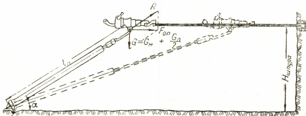
Рис. 1. Схема установки бурильного молотка на пневмоподдержке.
