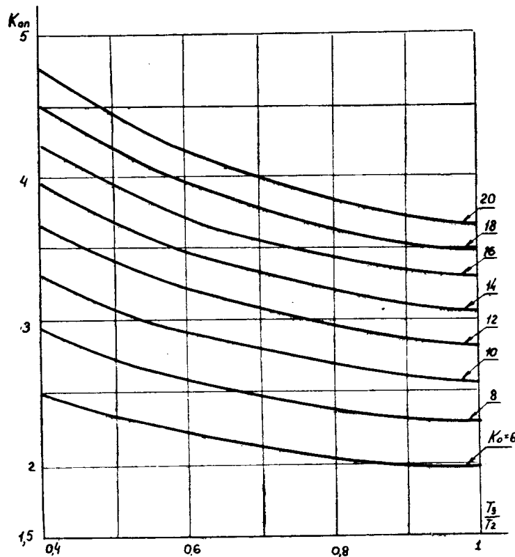
Рис. 2. К расчету оптимального коэффициента форсировки.
