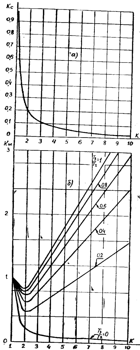
Рис. 1. Зависимость k_c и k_M от коэффициента форсировки.
