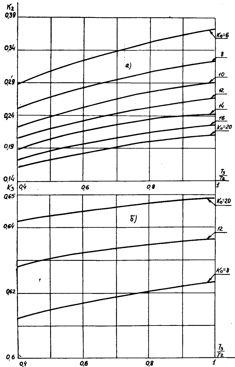
Рис. 3 Сравнение прерывистого возбуждения при k=k_{оп} с прерывистым возбуждением при k=1 и с постоянным возбуждением.
